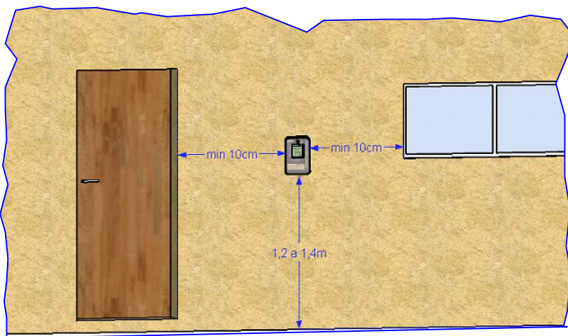
Detalle A
