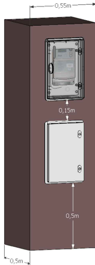
Dimensiones del pilar
