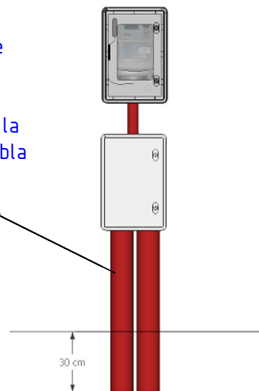
Detalle de los caños de acometida
