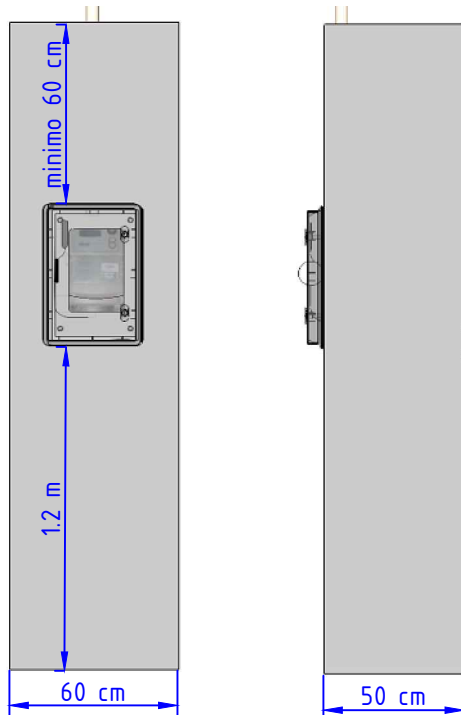
Dimensiones del pilar
