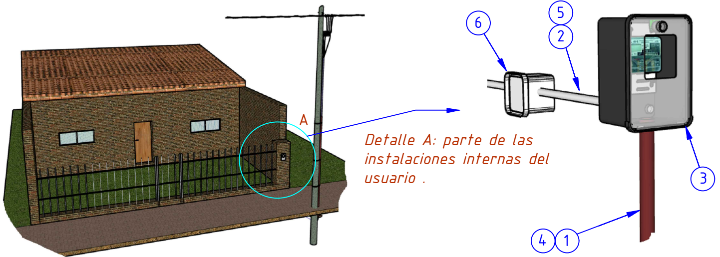
Vista general ejemplo de inmueble con alimentacion semisubterranea donde LE no coincide con LM
